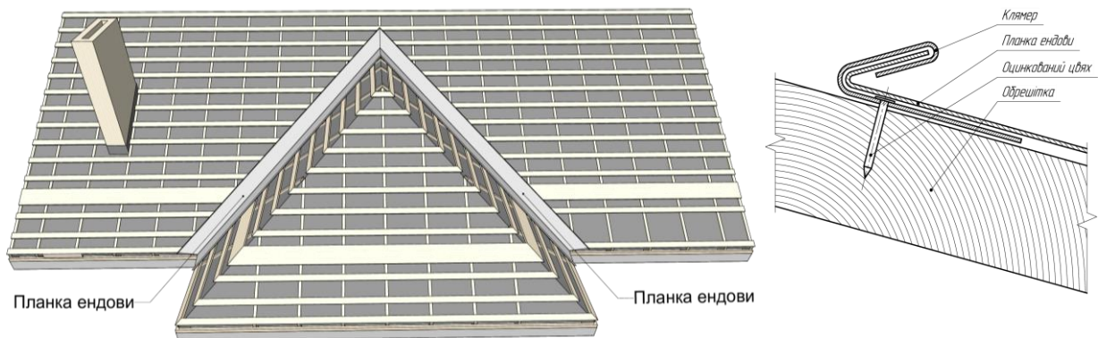
Рис.12 "Схема кріплення планки"
