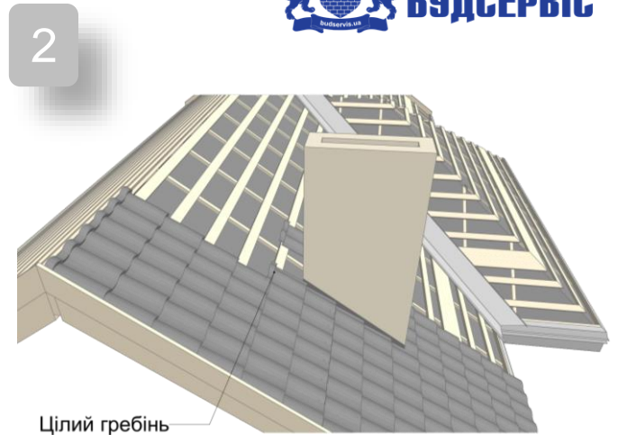
Рис.18 "Підрізка листів"
