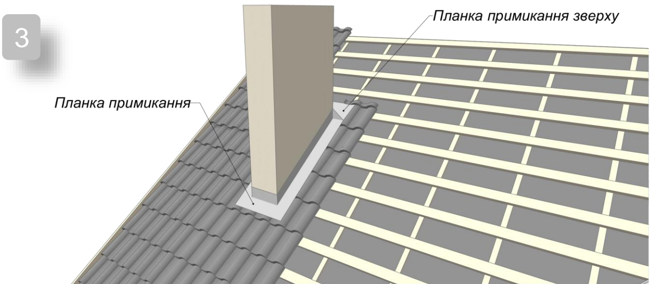
Рис.19 "Встановлення планок примикання"
