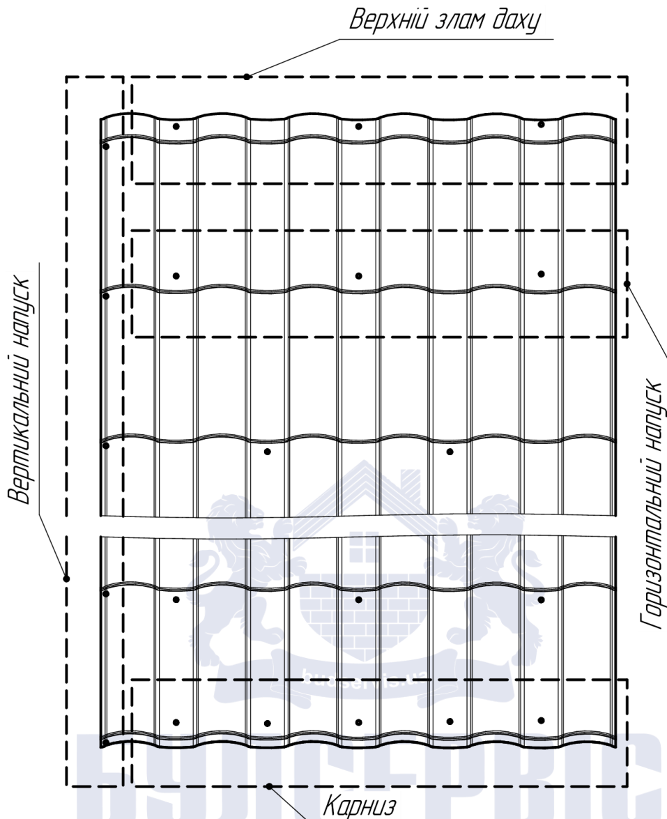
Рис.16 "Схема кріплення шурупів"
