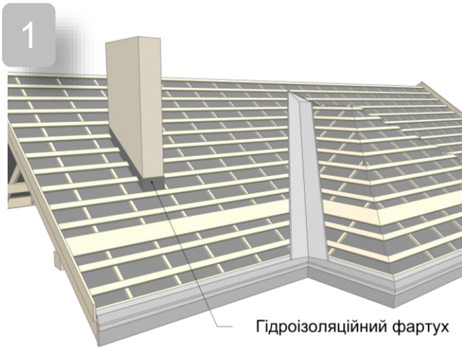
Рис.17 "Гідроізоляційний фартух"
